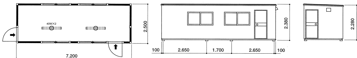
平面図
