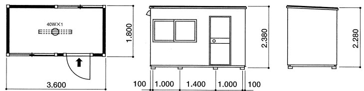
平面図
