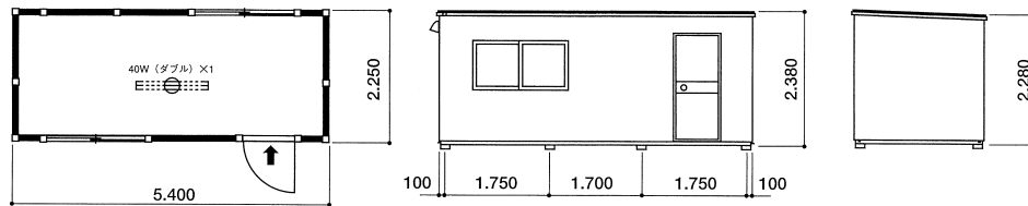
平面図
