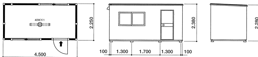
平面図
