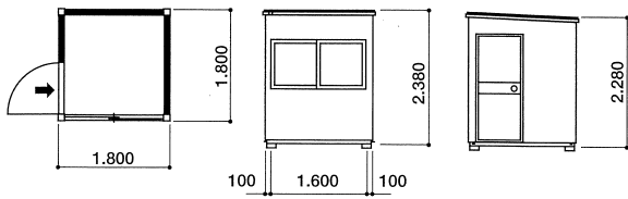
平面図
