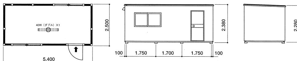
平面図
