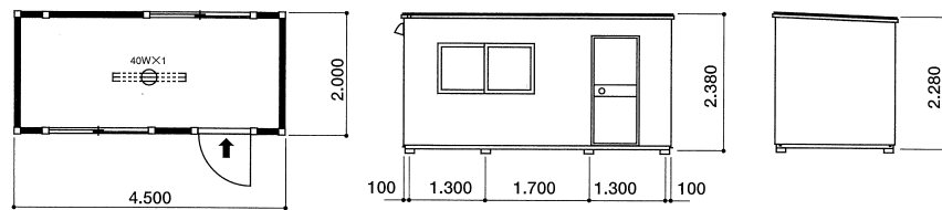
平面図
